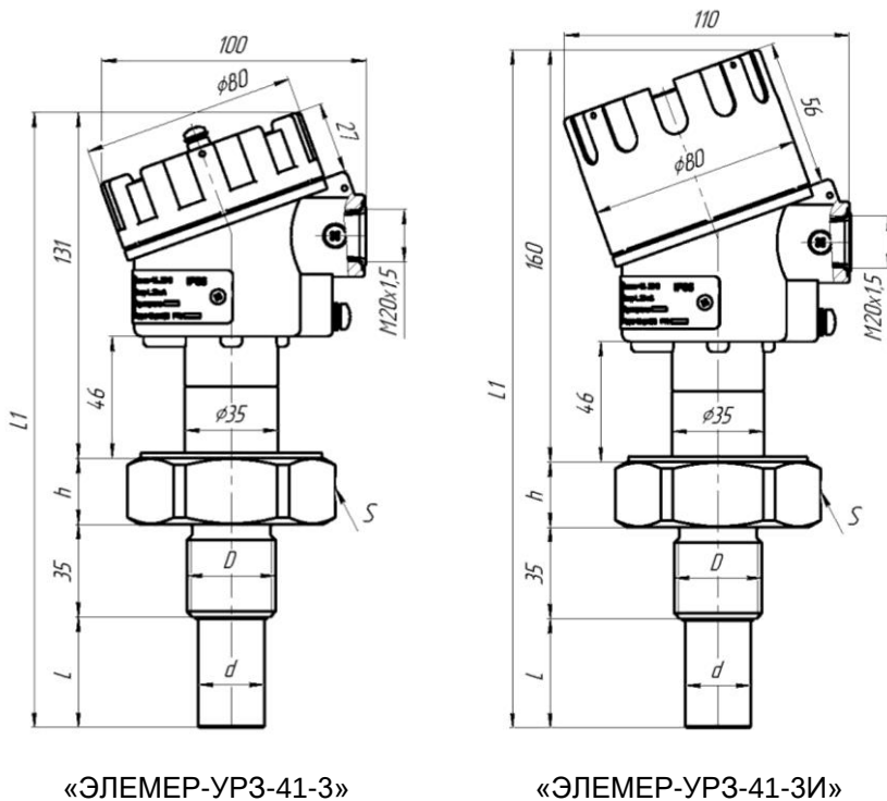
Рисунок А.1 – Габаритные размеры «ЭЛЕМЕР-УРЗ-41-3», «ЭЛЕМЕР-УРЗ-41-3И»
