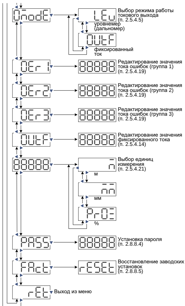
Рисунок 2.7 – Меню УРЗ-41-3И, УРЗ-41-4И
